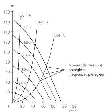
Fig. 6 : Fréquences prééglées
