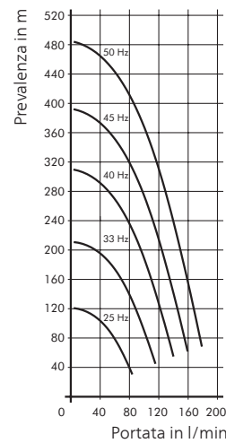
Sistemazione tandem attraverso convertitore di frequenza come comando a gruppo
